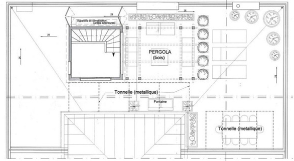
PLAN TERRASSE
