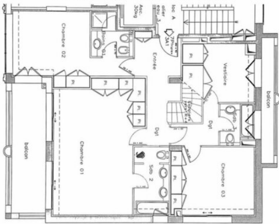
Plan modificatif - Appartements 3A1 + 4A1 - Niveau R+3
