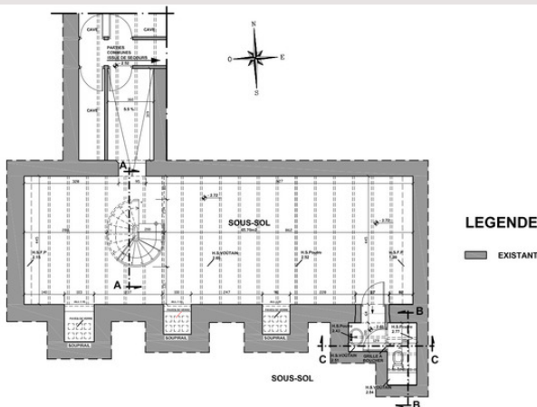
PLAN SOUS-SOL
