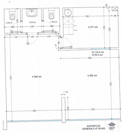
SUPERFICIE GENERALE 47.50 MQ
