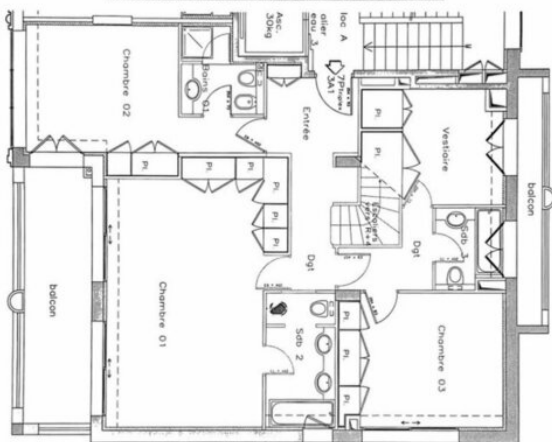
Plan modificatif - Appartements 3A1 + 4A1 - Niveau R+3
